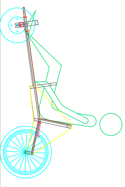
POSICIO DEL CONDUCTOR perfil explicatiu escala 1_20
